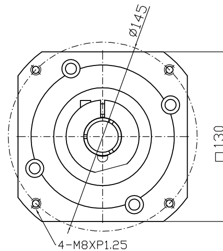
4-M8XP1.25
